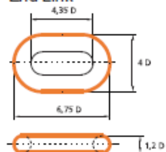
End Link
